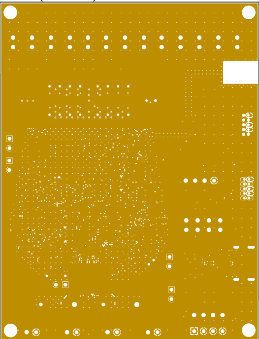
AHOR (Scale 1:1)
