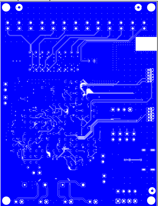
BOT (Scale 1:1)
