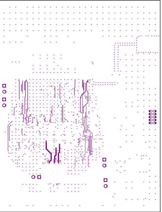
AVERT (Scale 1:1)
